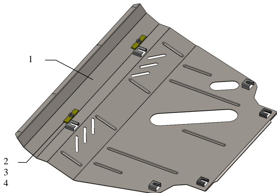
Schéma montáže krytu
